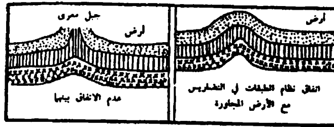
أثر التعرية في انقاض أطراف الأرض
